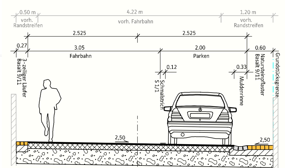
Regelquerschnitt B-B Brunnenstraße M 1:50
